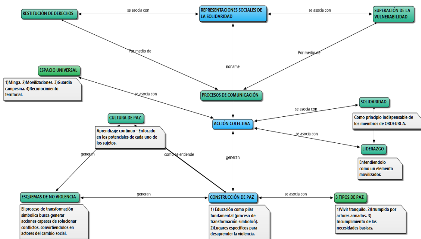
Figura 1. Red semántica
